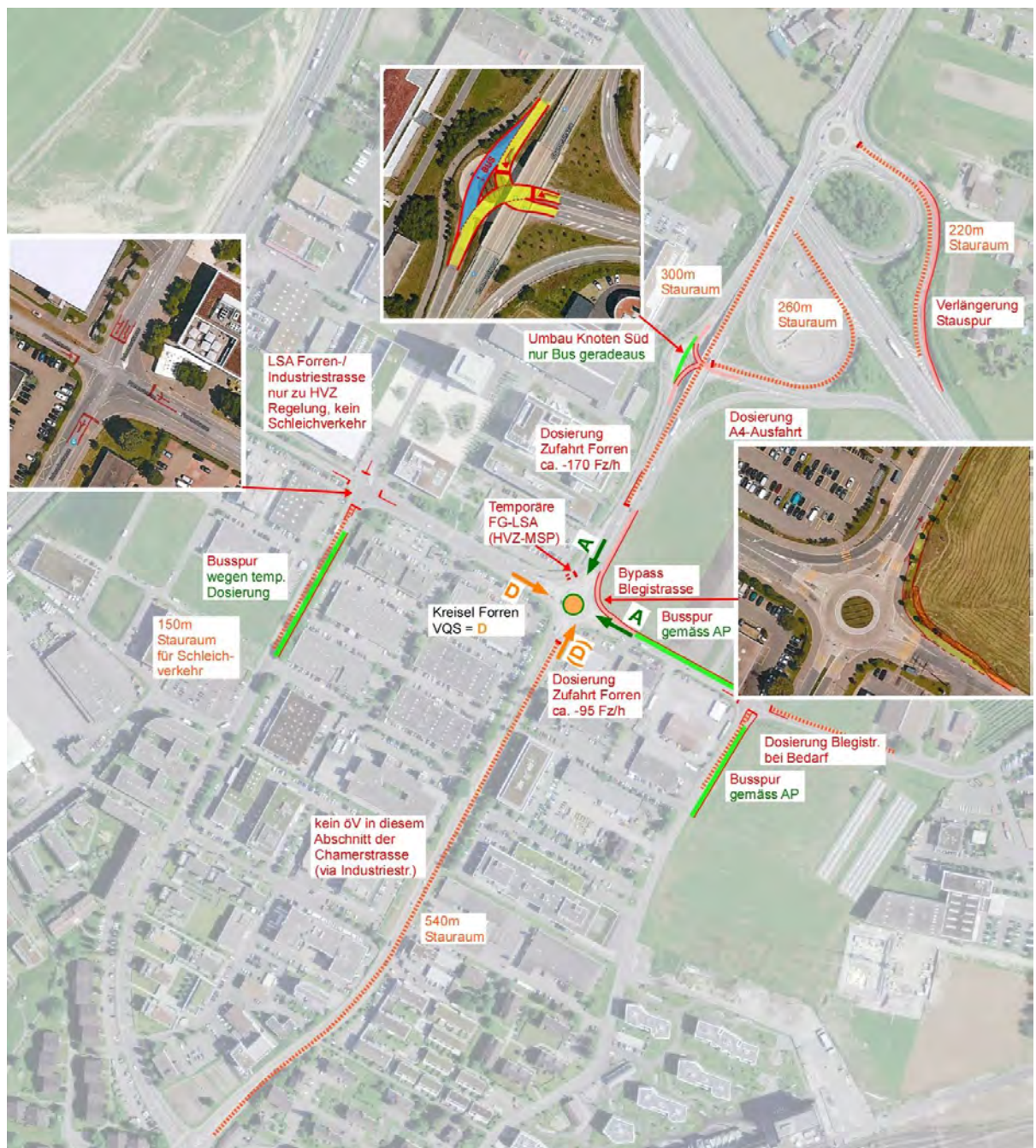
Abbildung 26 Massnahmenkonzept für Verkehrsmanagement Rotkreuz Industrie/Forren
