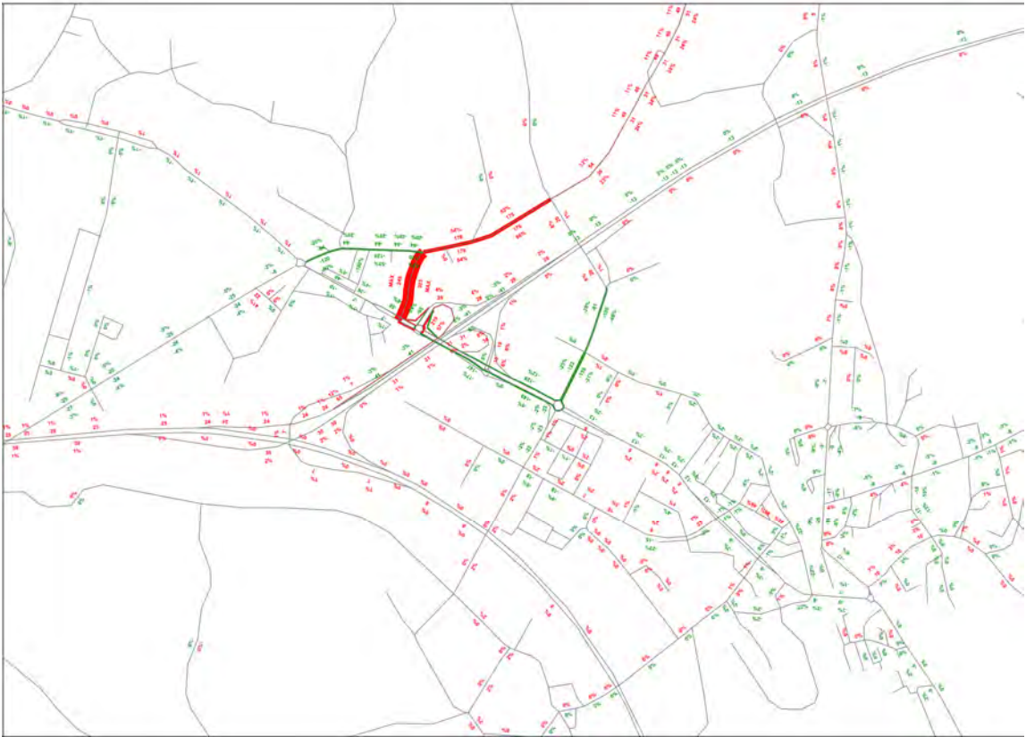
Differenzen Massnahme R3 MINUS Referenzzustand MSP 2030 [Mfz/h; %]
