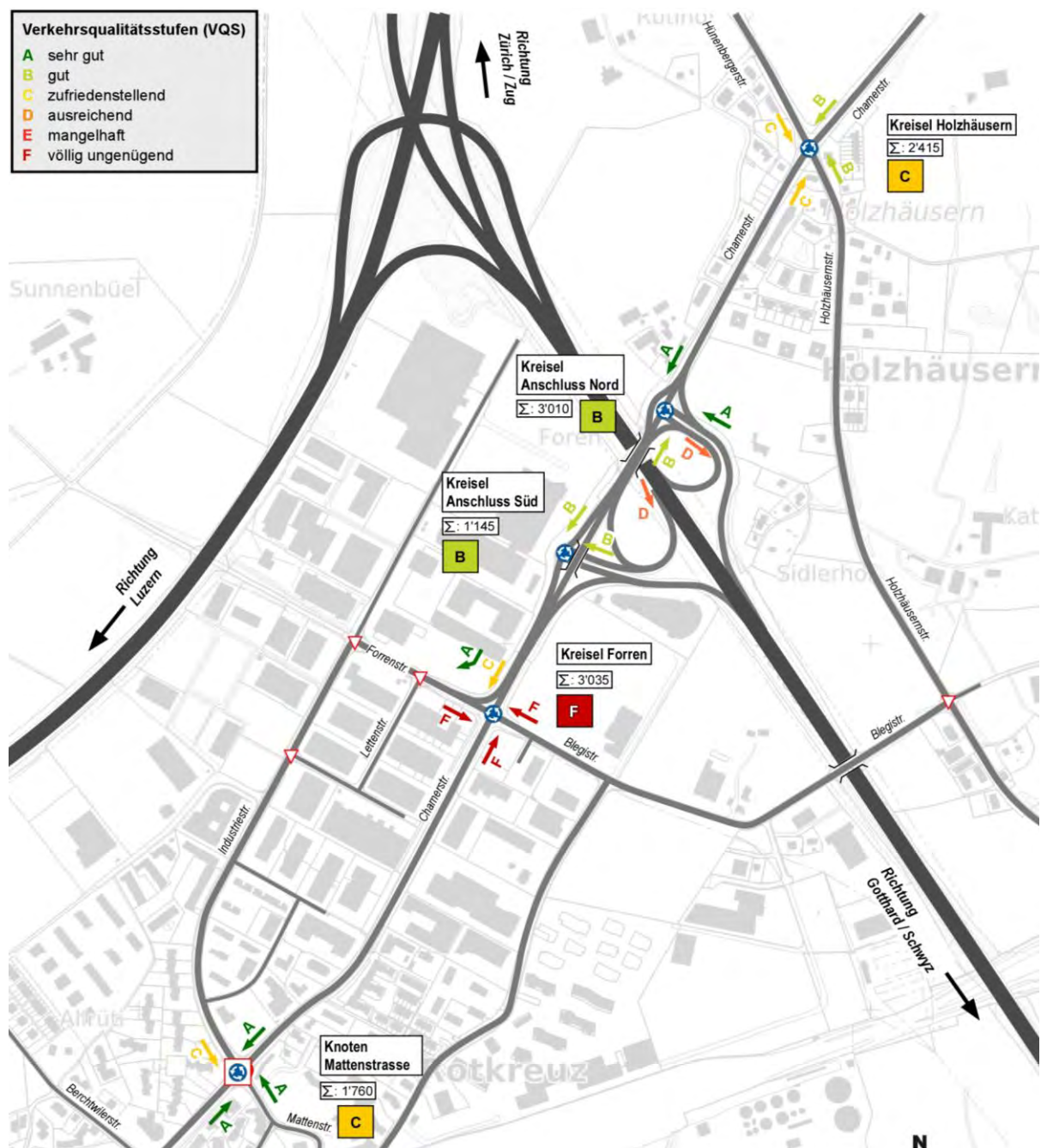
Abbildung 20 Auslastungen Prognosezustand 2030 Abendspitze
