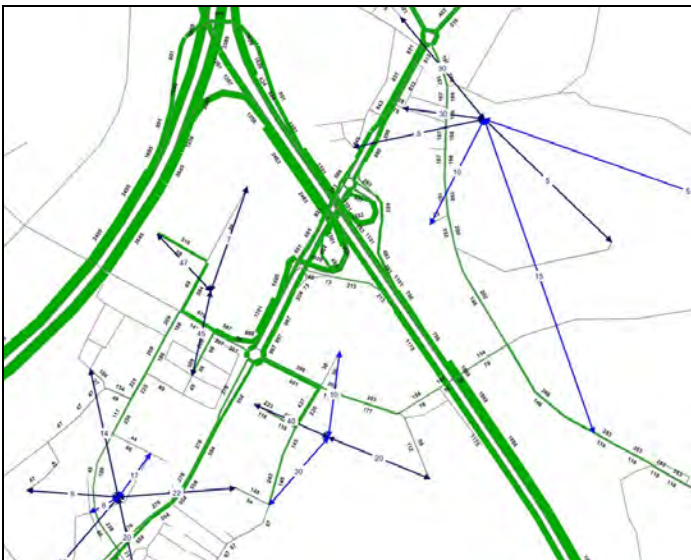
Zonenanbindungen und veränderte Netzcodierung (Attribute) für Zustand 2015
