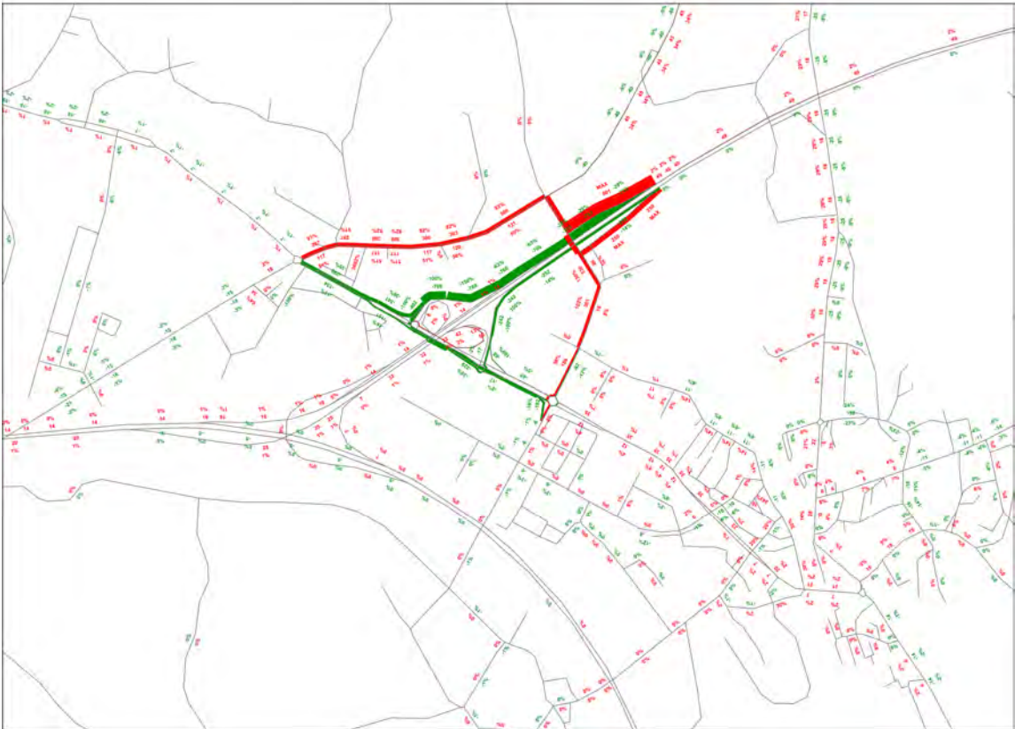
Differenzen Massnahme A3 MINUS Referenzzustand MSP 2030 [Mfz/h; %]
