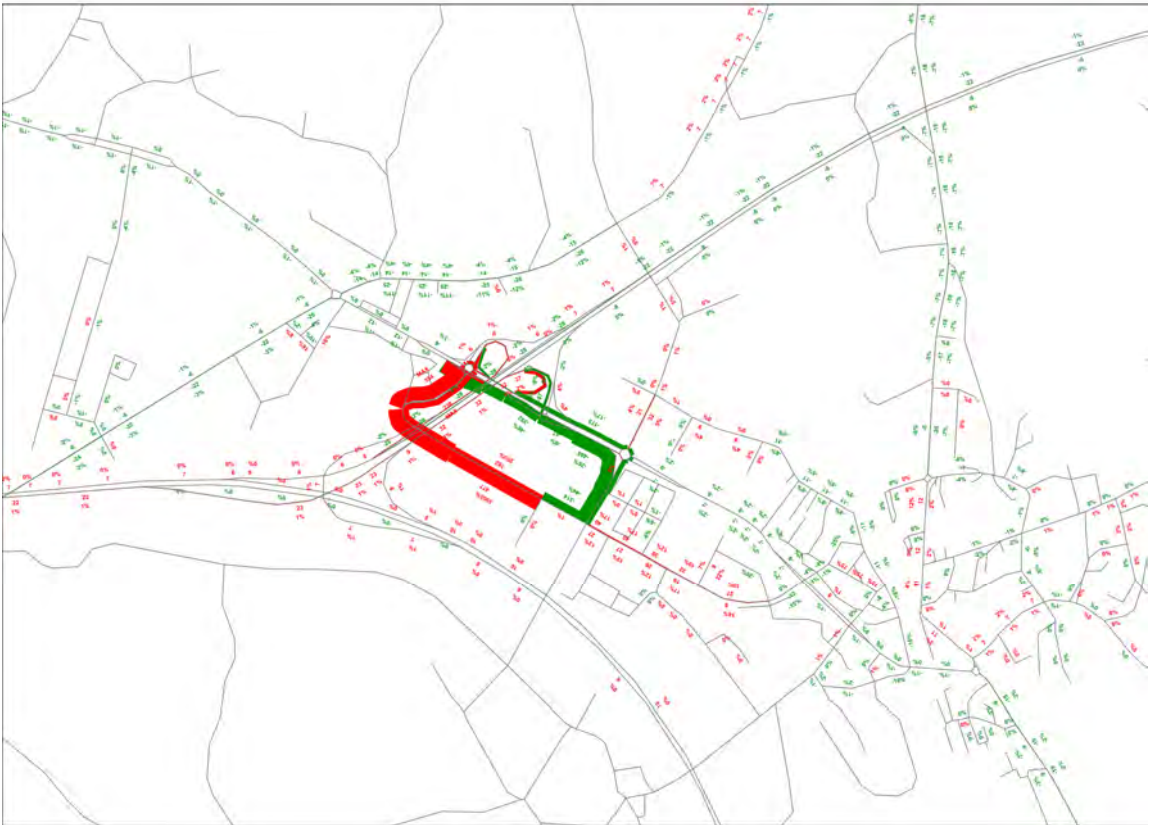
Differenzen Massnahme E1 MINUS Referenzzustand MSP 2030 [Mfz/h; %]
