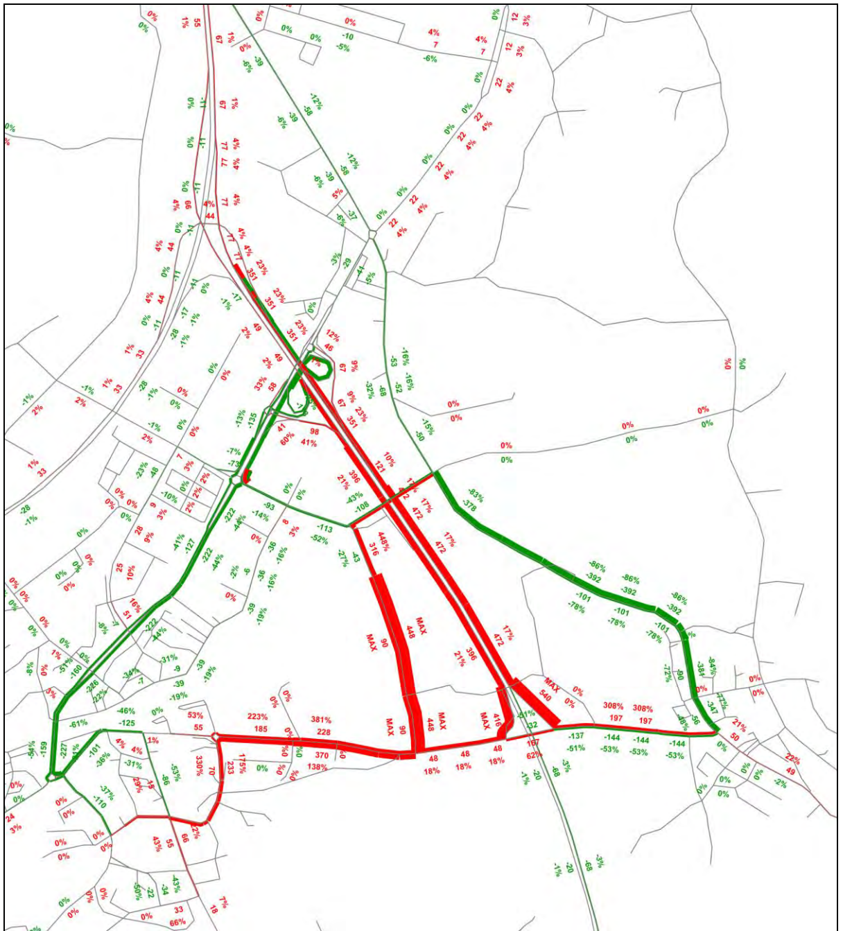
Abbildung 44 Belastungsänderungen mit Ostumfahrung in der Morgenstipfe 2030 [Mfz/h] bzw. [%]
