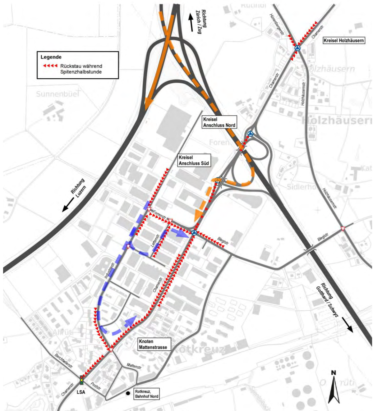
Abbildung 13 Problemplan Abendspitze Ist-Zustand
