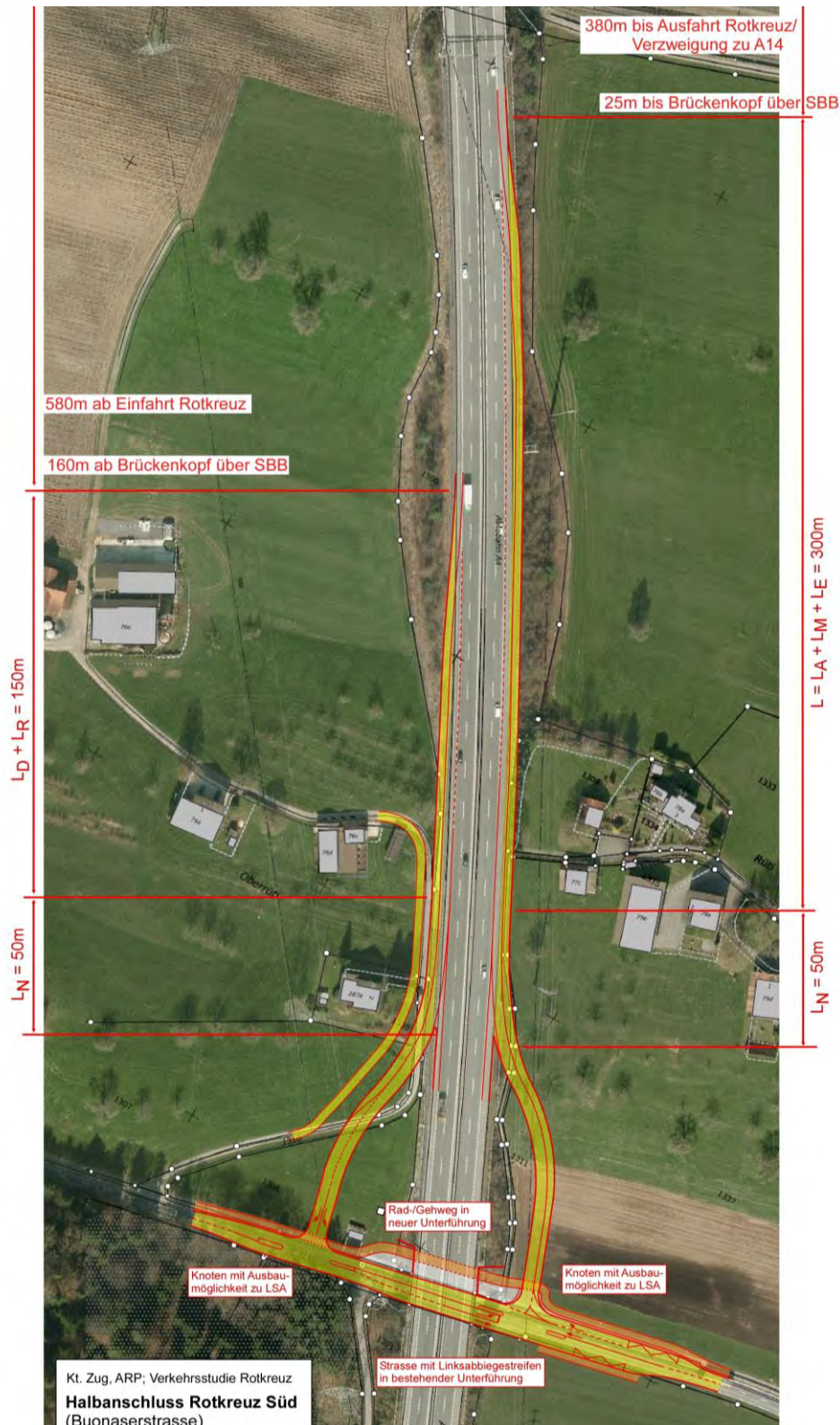
Abbildung 38 Planskizze Halbanschluss A4 Buonaserstrasse
