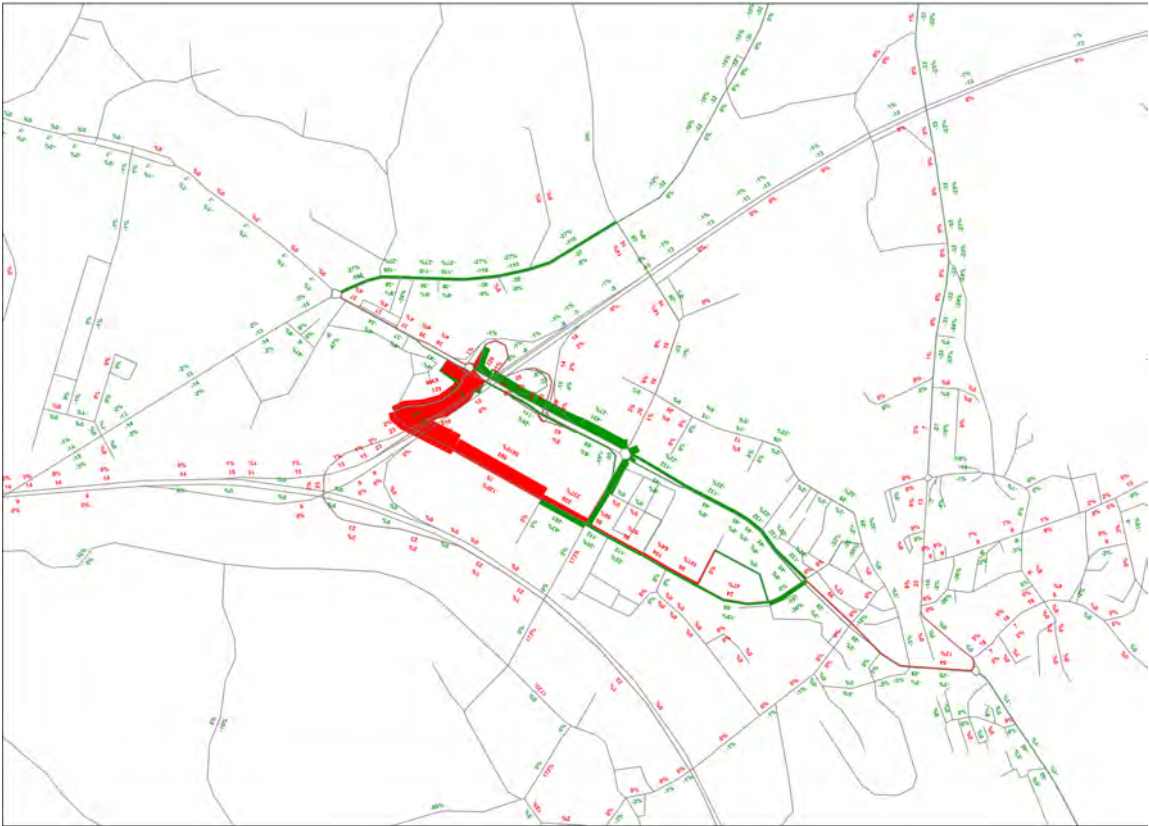
Differenzen Massnahme E1 MINUS Referenzzustand ASP 2030 [Mfz/h; %]
