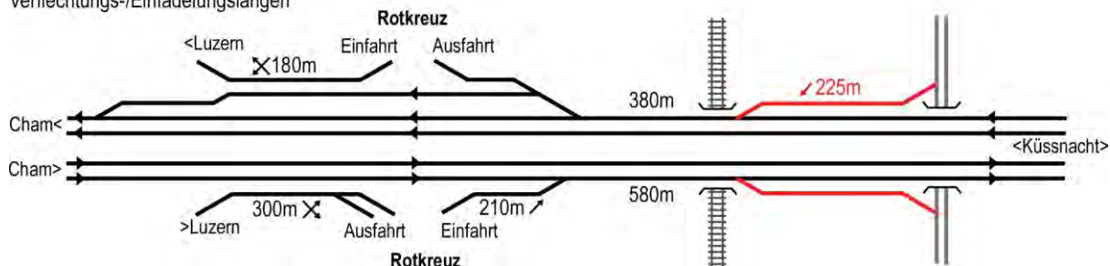
Abbildung 39 Fahrstreifenschema auf der A4 im Bereich Anschluss Rotkreuz mit Verflechtungslängen
