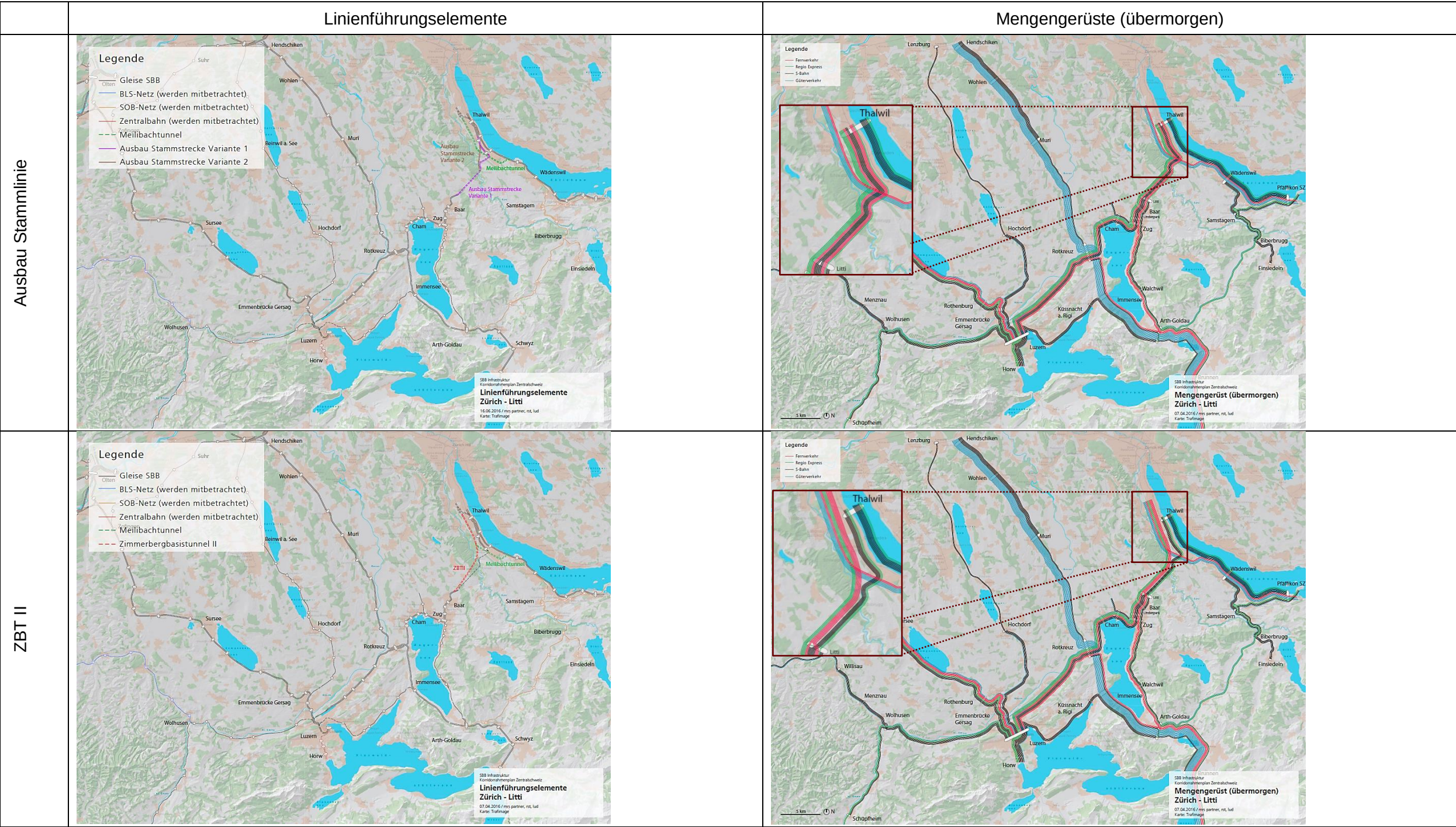
Abb. 43: Variantenfächer Zürich–Litti
