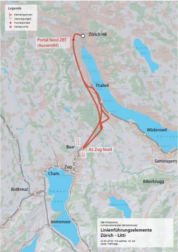
Abb. 50: Linienführungselemente im Abschnitt Zürich–Litti
