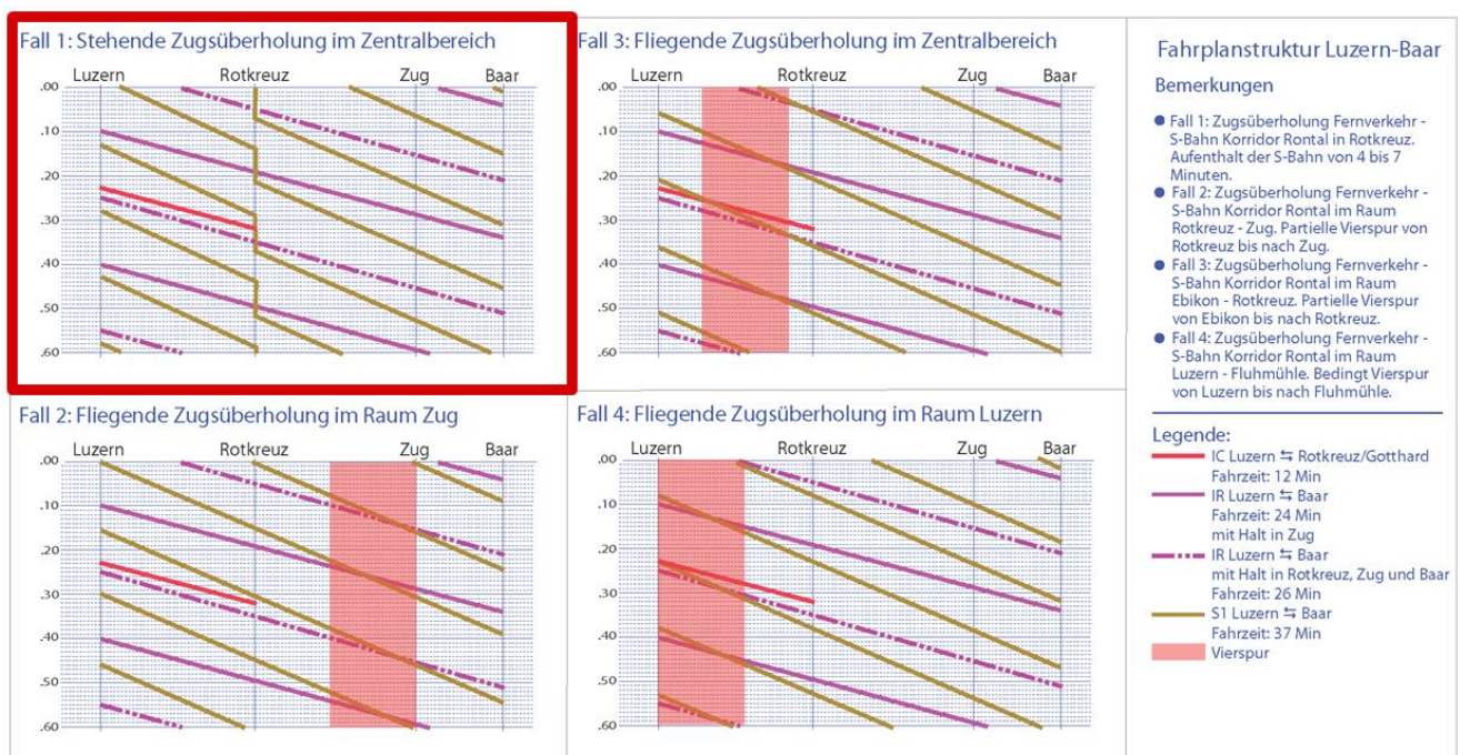
Abb. 63: Lösungsansätze für die Zugsüberholungen Luzern–Baar
