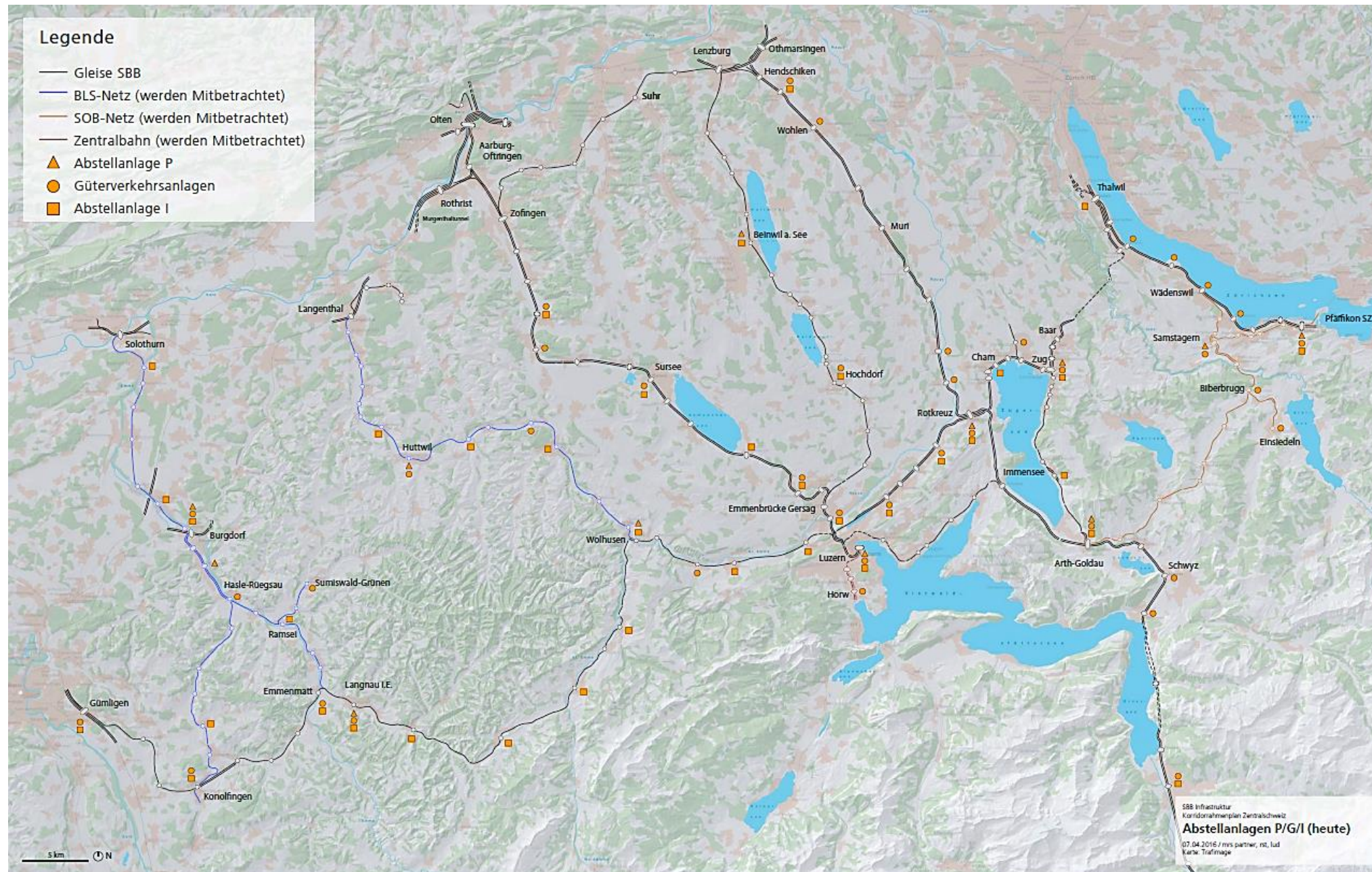
Abb. 16: Abstellanlagen Personen-/Güterverkehr/Infrastruktur
