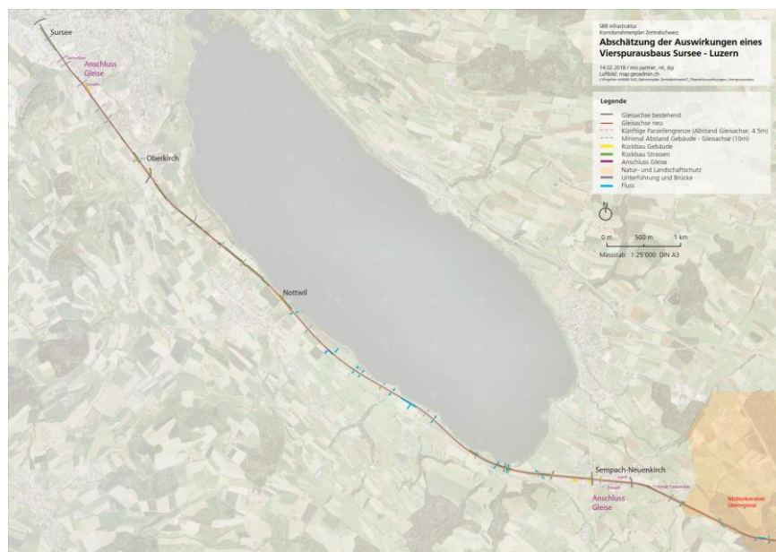
Abb. 68: Abschätzung der Auswirkungen eines Vierspurausbaus Sursee–Luzern (Teil 1)
