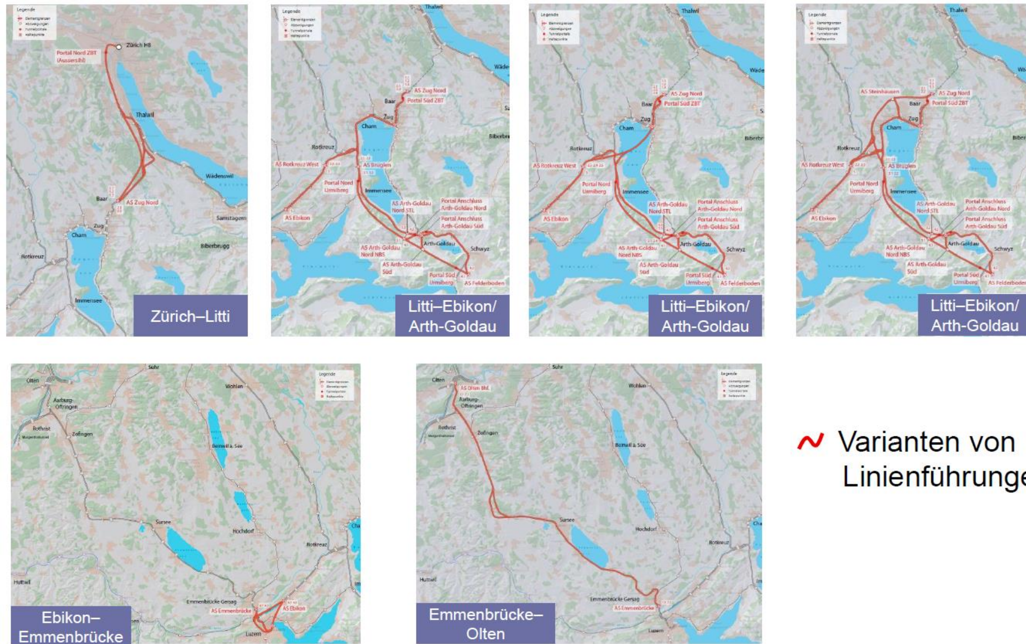
Abb. 3: Linienführungselemente
