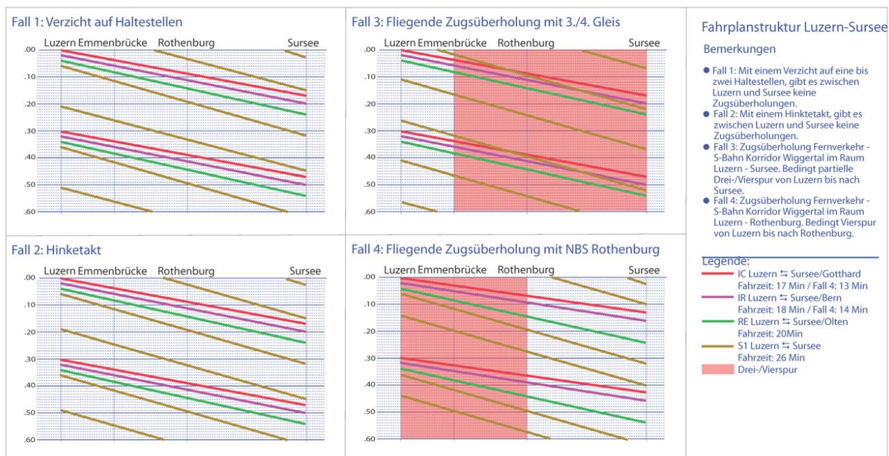
Abb. 64: Lösungsansätze für die Zugsüberholungen Luzern–Sursee
