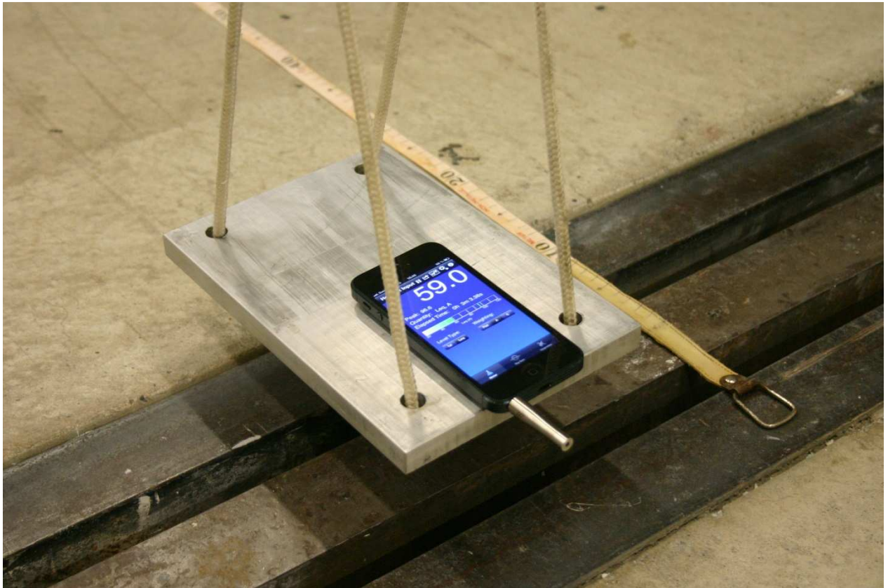
Abbildung 4: Pendelplatte in Ruhelage mit installiertem Smartphone und externem Mikrofon ohne Windschirm.
