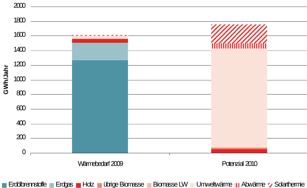
Abbildung 1: Heutiger Wärmebedarf im Kanton Zug aufgeteilt nach Energieträgern sowie Potenzial an lokalen erneuerbaren Energien zur Wärmergewinnung.
